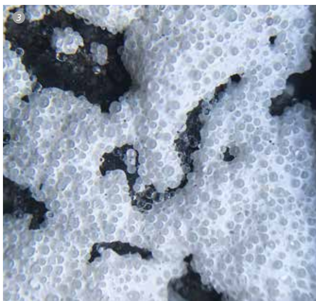
Mikrokulki szklane na strukturalnym oznakowaniu poziomym
