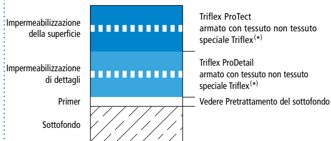
Struttura del sistema – Dettaglio B
