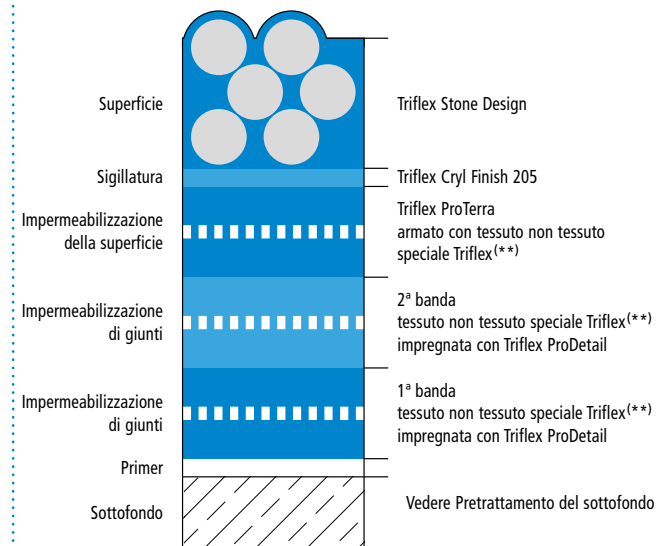
Struttura del sistema – Dettaglio C
