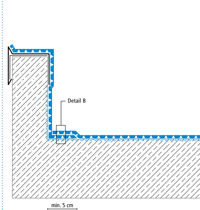
Parapet edge finishing
