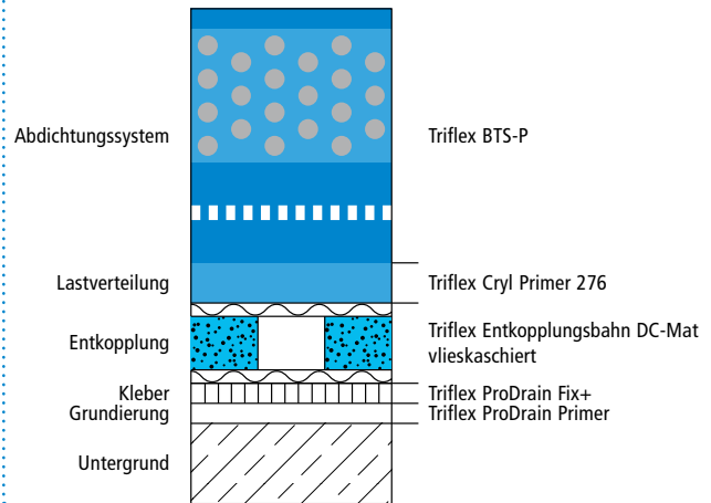
Systemaufbau – Detail A
