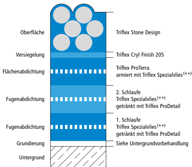
Systemaufbau – Detail C
