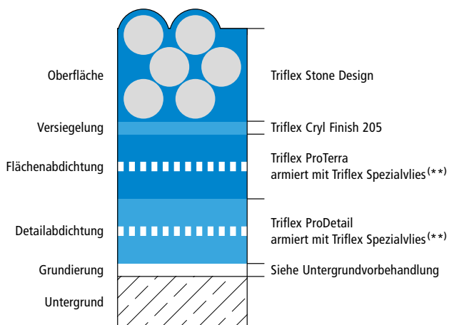
Systemaufbau – Detail B
