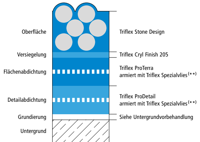
Systemaufbau – Detail B
