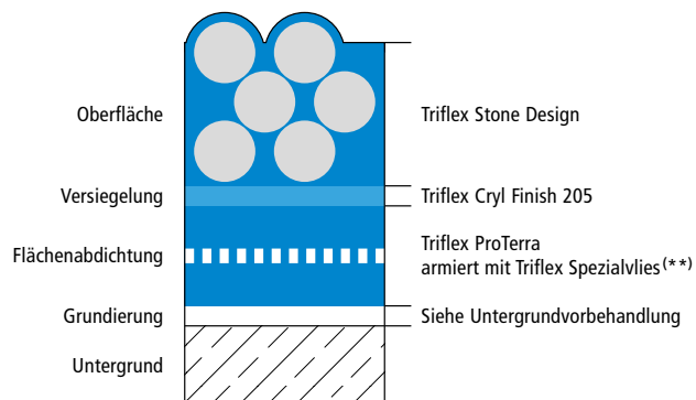
Systemaufbau – Detail A
