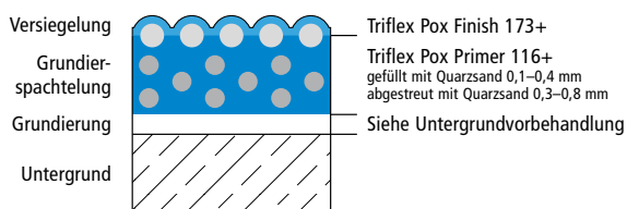
Systemaufbau, Variante 2 – Detail B
